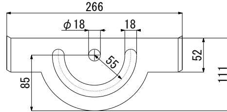
<取付け部寸法>
